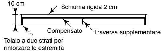
Schema costruttivo alleggerito
